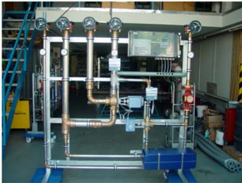
Gössi-Mat Anlage mit thermischer Desinfektion
